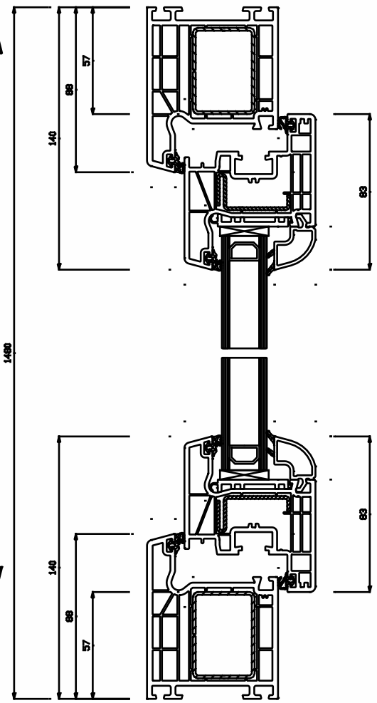
Schnitt S1(5:1)
