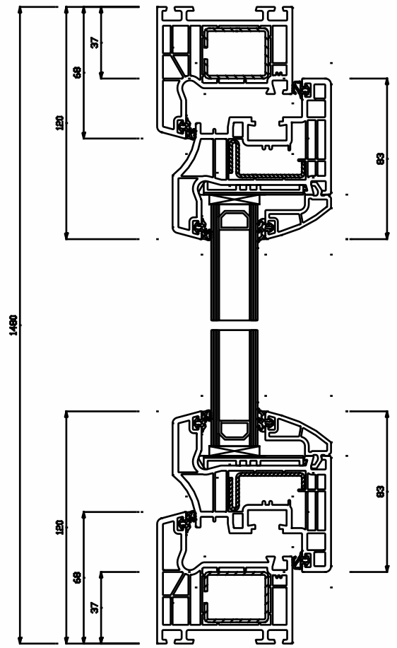
Schnitt S1(5:1)
