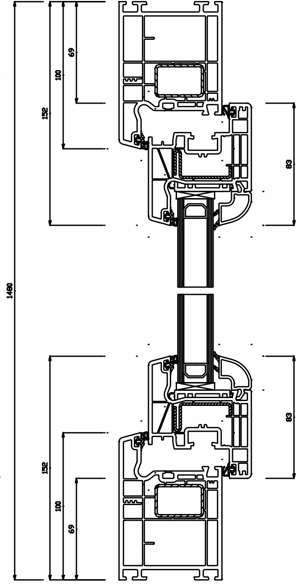
Schnitt S1(5:1)
