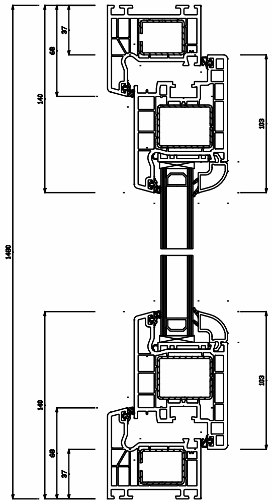
Schnitt S1(5:1)
