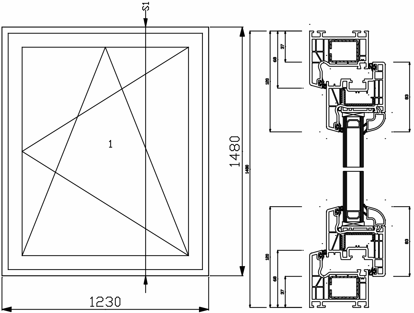
Schnitt S1(5:1)
