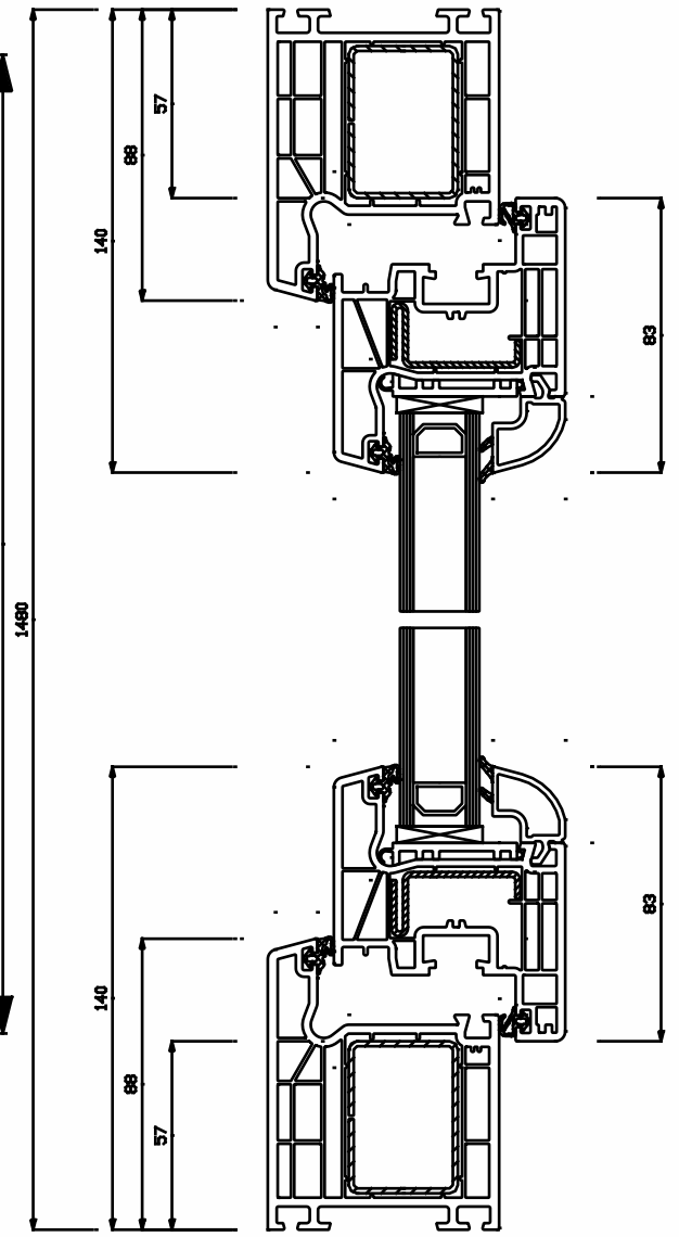
Schnitt S1(5:1)
