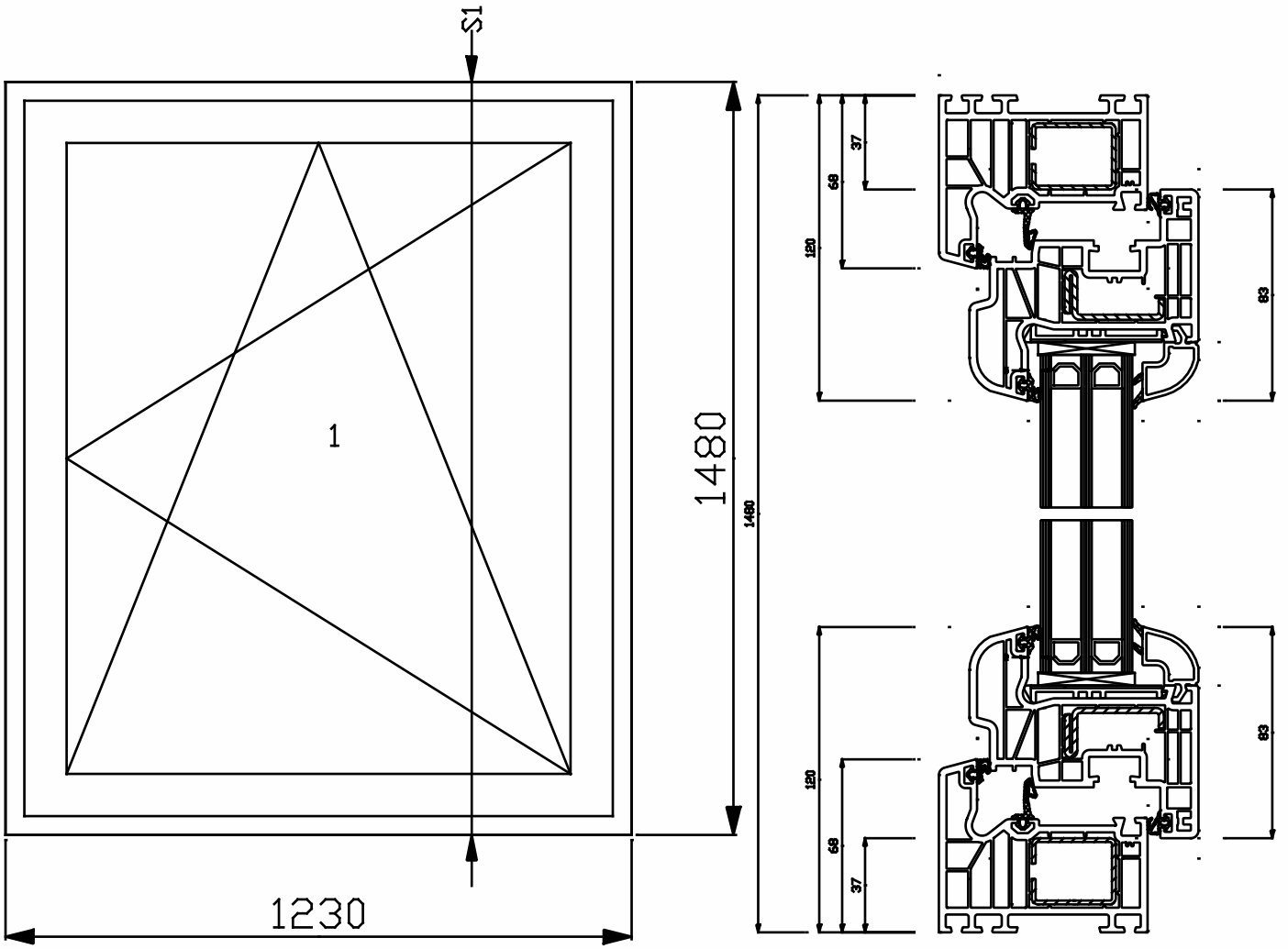
Schnitt S1(5:1)
