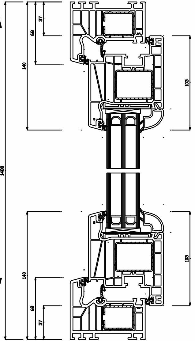
Schnitt S1(5:1)
