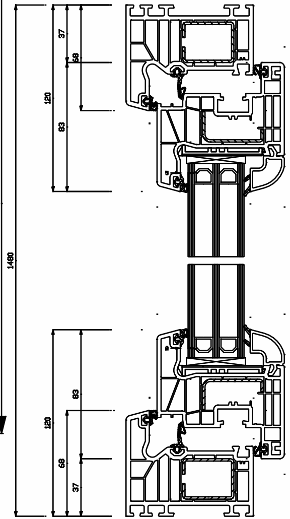
Schnitt S1(5:1)
