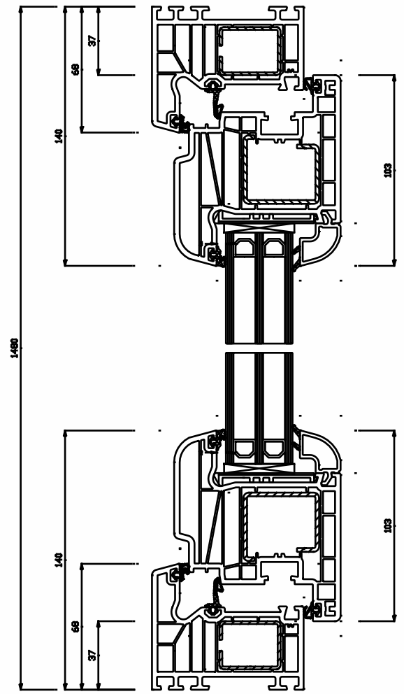
Schnitt S1(5:1)
