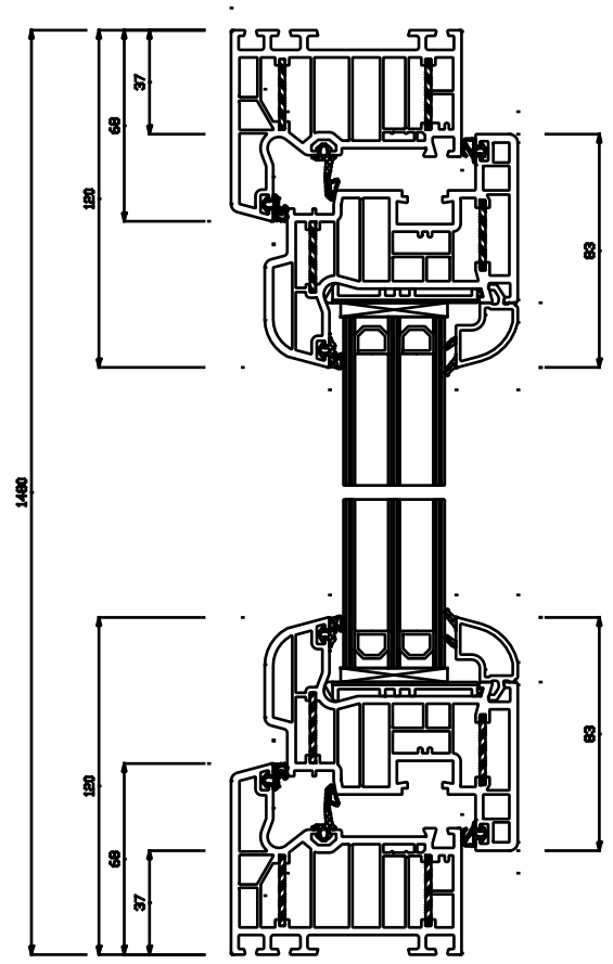
Schnitt S1(5:1)
